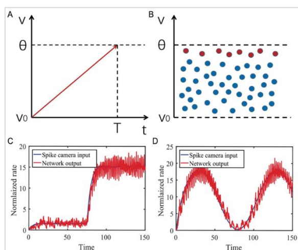
图3.4 兴奋-抑制平衡网络对输入变化的快速响应。(A) 单神经元接受“干净”输入的整合发放过程，神经元的整合时间由神经元的膜电位时间常数决定。(B) 神经元群的膜电位分布使得神经元群可以快速的响应外部刺激，红色的点表示接近发放阈值的神经元，其可以快速地响应外部刺激变化。(C, D) 兴奋-抑制平衡的神经网络对不同的，随时间变化的刺激可以快速响应，其中蓝色的曲线为脉冲摄像头的输入，红色的曲线为神经元群的输出[6]。
